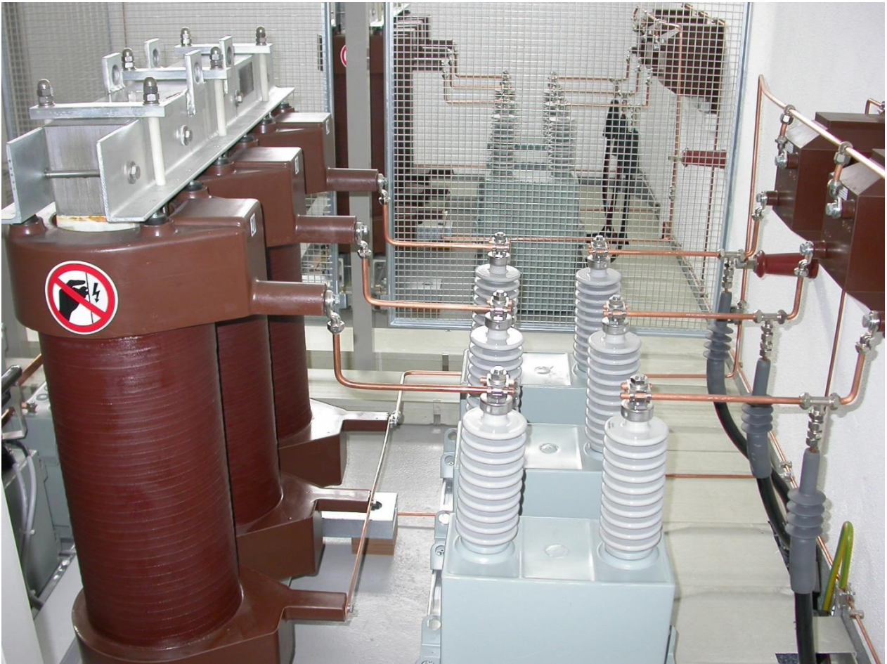
Bild: Ankoppelung Rundsteueranlage
